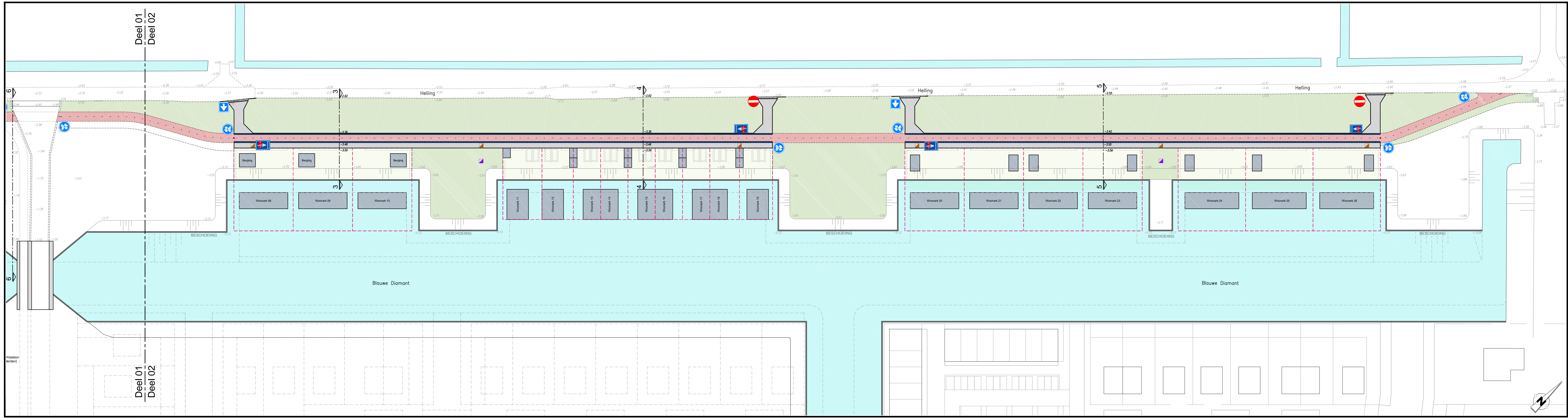
Terreininrichting, deel 2 schaal 1:500
