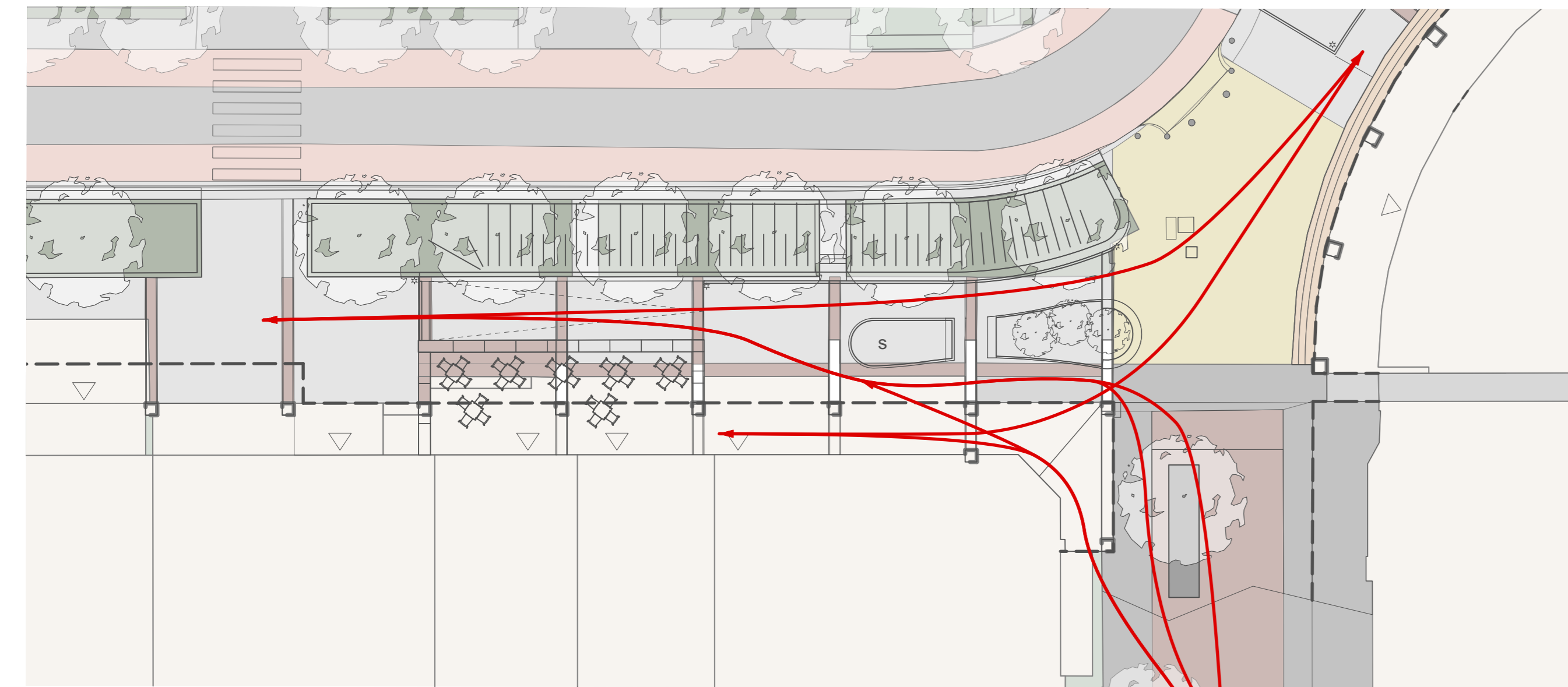
5 Definitief ontwerp met looplijnen Schaal: 1:200
