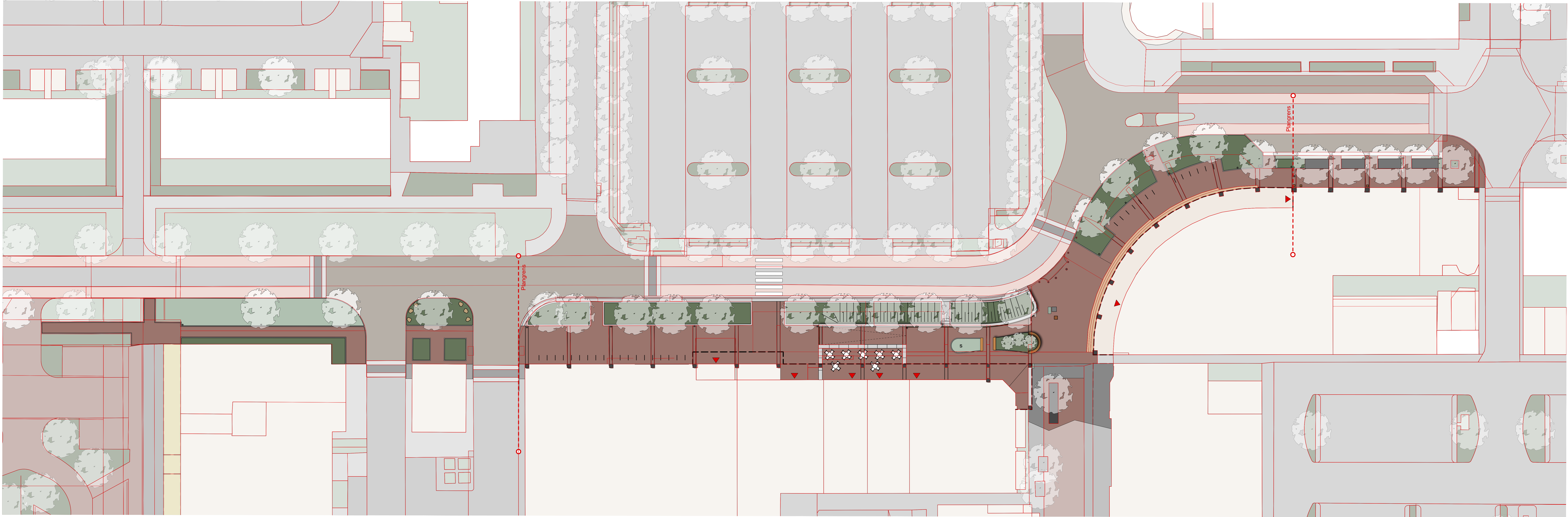
4 Definitief ontwerp met huidige topo in rood Schaal: 1:200
